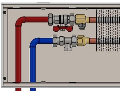
Рисунок 19-в. Угловое - со стороны помещения.
