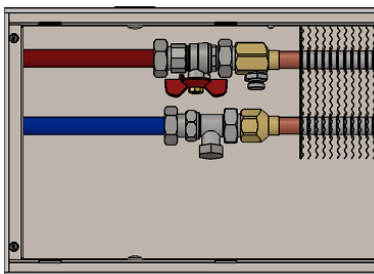
Рисунок.19-а.Прямое- без использования гибких шлангов.
