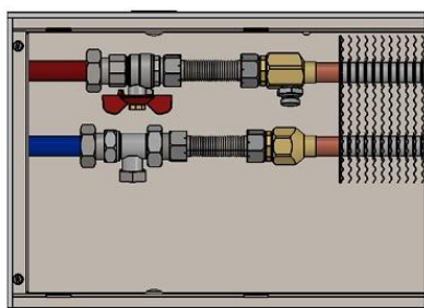
Рисунок 19-б. Прямое - используя гибкие шланги.
