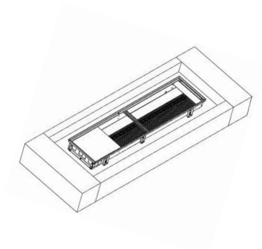
Рисунок 10. Удалите на корпусе заглушки, необходимые для подсоединения по воде.
