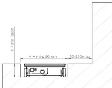
Рисунок 4. А - максимальная ширина корпуса конвектора (L - длина конвектора); Н - высота корпуса конвектора (без выравнивающих ножек). Рекомендуемые размеры для монтажа: В + 50 мм; L + 50 мм; Н + 10 мм, расстояние до стены 50-350 мм.
