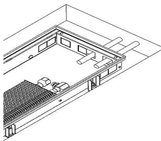
Выровняйте конвектор в горизонте с помощью юстировочных винтов, рис. 13а.
