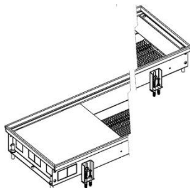
Рисунок 8. Поставьте конвектор на место монтажа. Сделайте отметки в местах крепления к полу, удалите конвектор для сверления отверстий.
