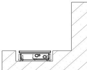
Рисунок 2. Монтаж конвектора в качестве основного источника тепла, с теплообменником расположенным со стороны помещения.
