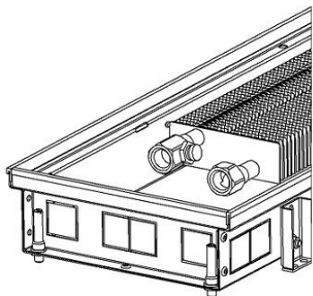
Рисунок 7. Вкрутите установочные винты для последующей фиксации анкерных ножек.
