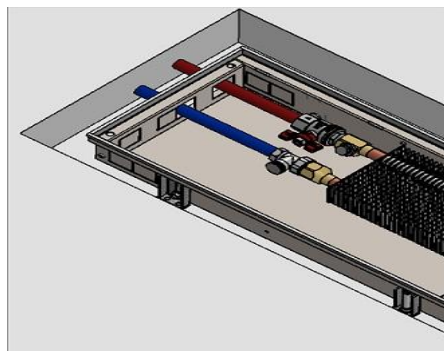
Рисунок 14. Подключение подачи и возврата теплоносителя
