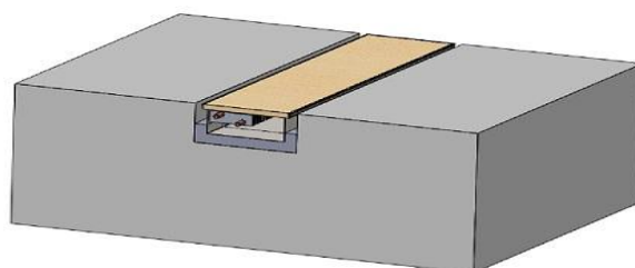
Рисунок 17. Не менее 1/3 высоты конвектора тщательно заливают жидким цементным раствором для снижения передачи звука.
